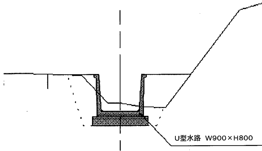
標準断面図
