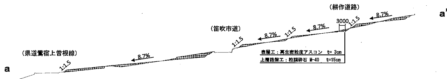
標準断面図
