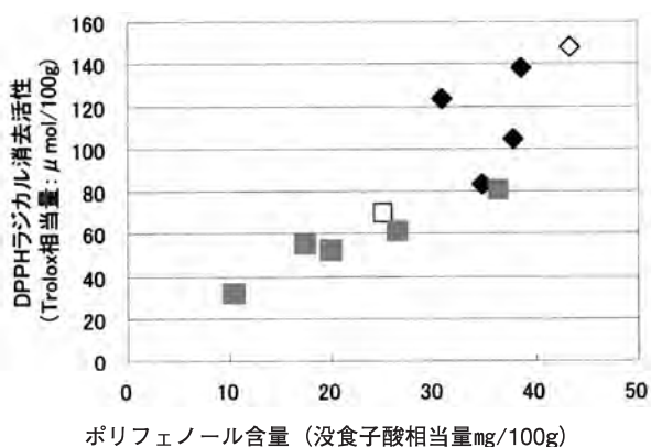
図6 ジャガイモの抗酸化活性と及びポリフェノール含量 (■: 可食部 (皮無) 試料, ◆: 皮付試料, □◇: おちあいいも)
