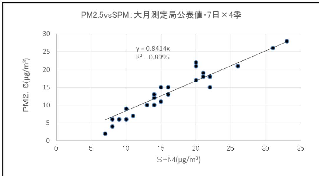
図 9-1-8 大月測定局における PM2.5 と SPM の関係
