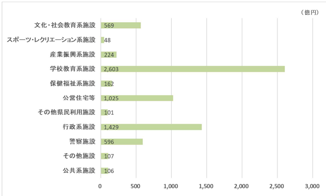
図 1 1 長寿命化型 施設類型別（中分類）更新費等の見込額（50年間）
