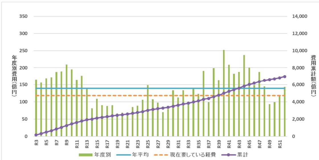
図10 公共建築物（長寿命化型）更新費等の見込額
