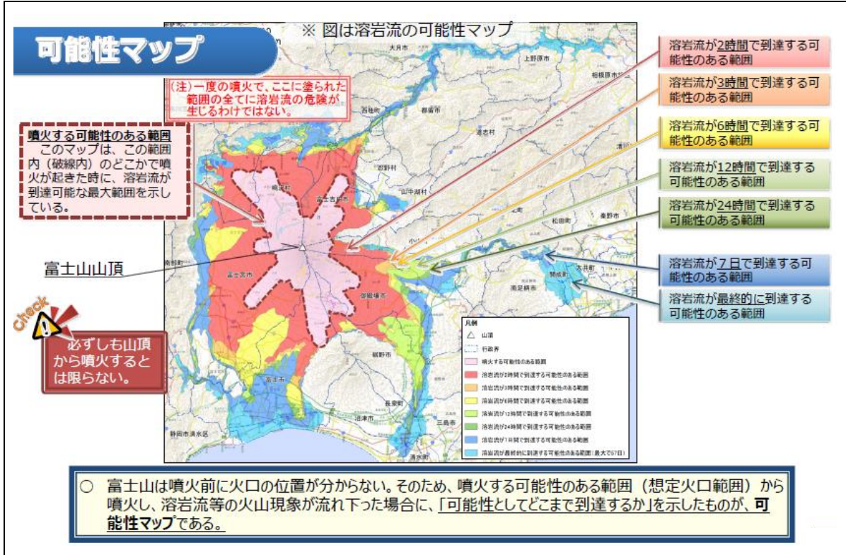
図 6.4-3 マップの図解例(溶岩流の可能性マップ)
