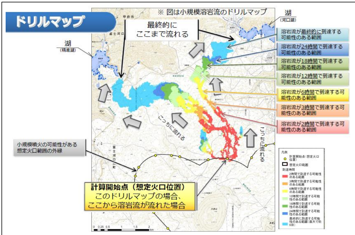
図 6.4-2 マップの図解例(溶岩流のドリルマップ)
