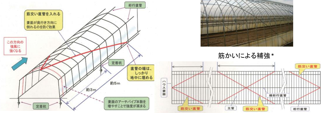
筋かいによる妻面の補強方法事例
