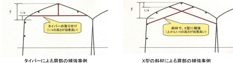
タイバーによる肩部の補強事例
