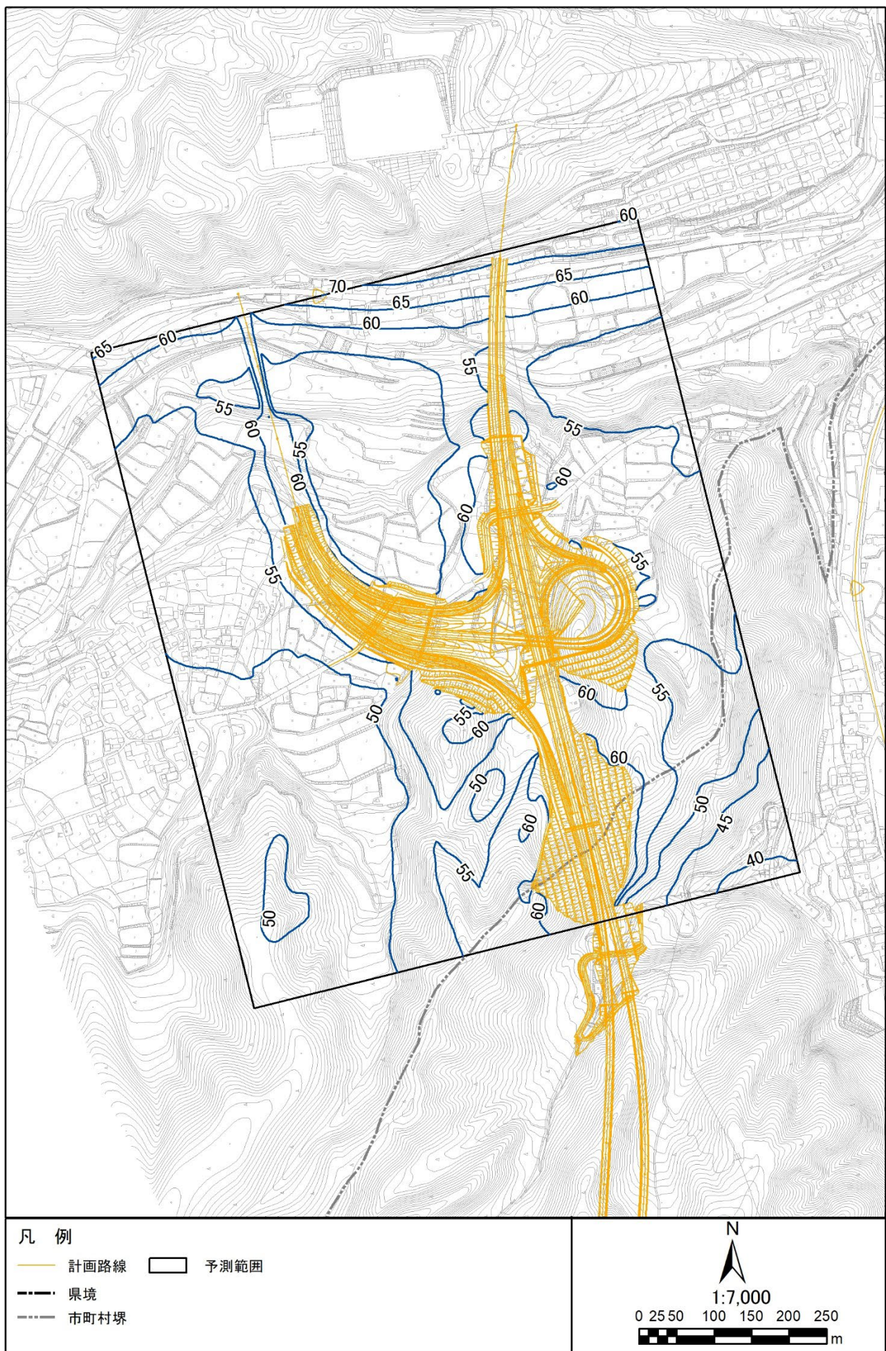
図 3.1-2 (22) 環境保全措置後の騒音分布図 (N9. 佐久穂町千代里) 地上 4.2m 昼間
