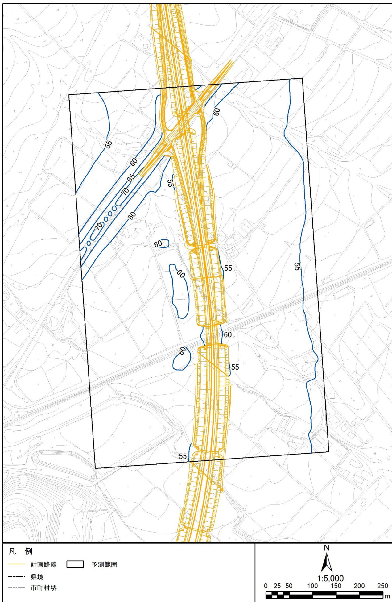
図 3.1-2 (5) 環境保全措置後の騒音分布図 (N1. 南牧村野辺山 1) 地上 1.2m 昼間
