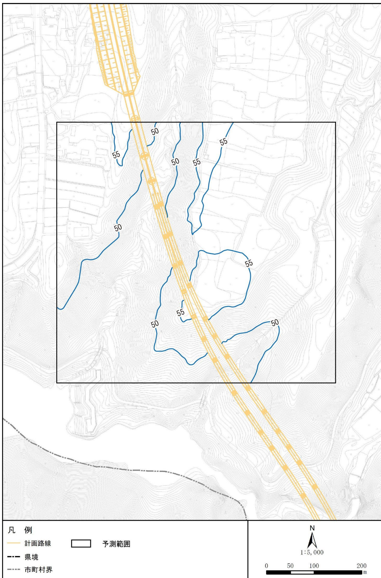
図 3.1-1 (11) 騒音分布図 (Y7. 高根町清里 1) 地上 1.2m 夜間
