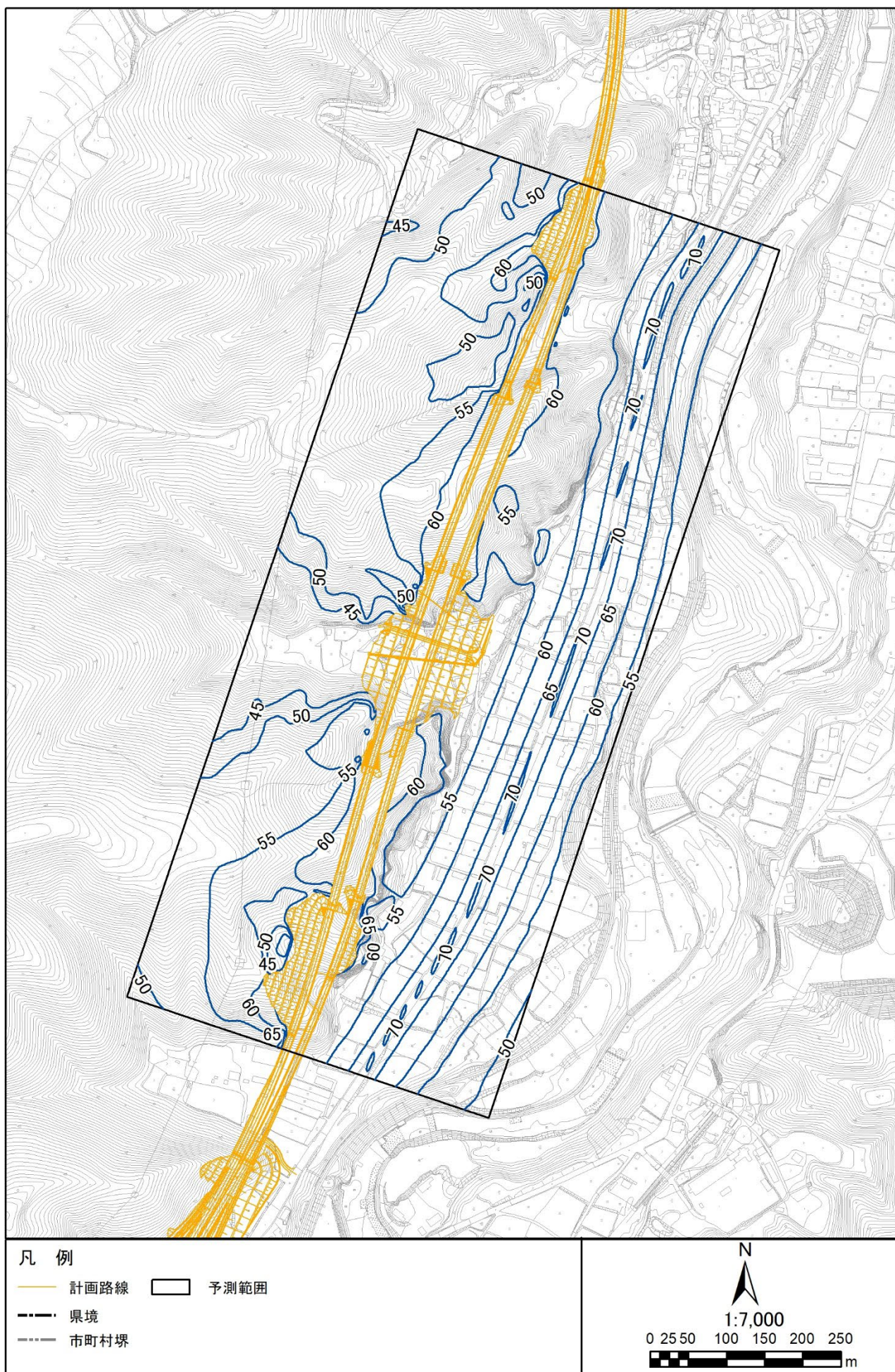
図 3.1-2 (18) 環境保全措置後の騒音分布図 (N6. 小海町豊里鎰掛1) 地上 4.2m 昼間
