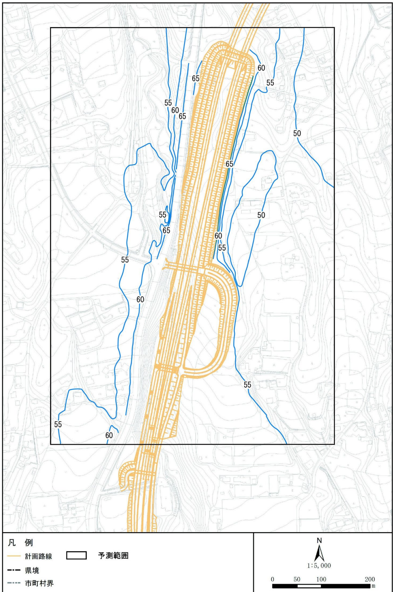
図 3.1-2 (1) 環境保全措置後の騒音分布図 (Y9. 高根町清里 3) 地上 1.2m 昼間
