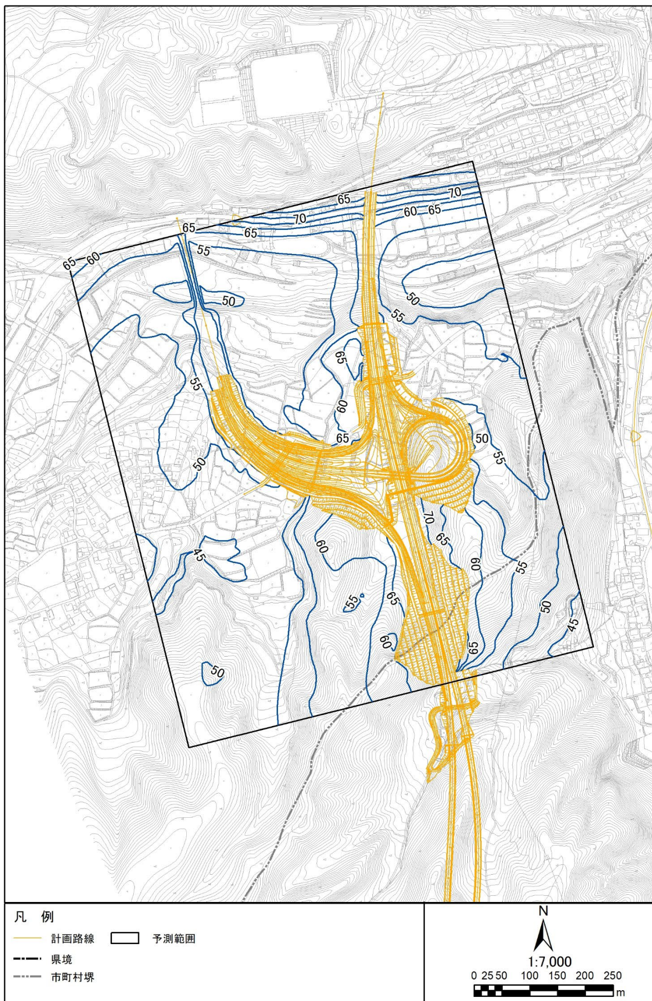
図 3.1-1 (33) 騒音分布図 (N9. 佐久穂町千代里) 地上 1.2m 昼間
