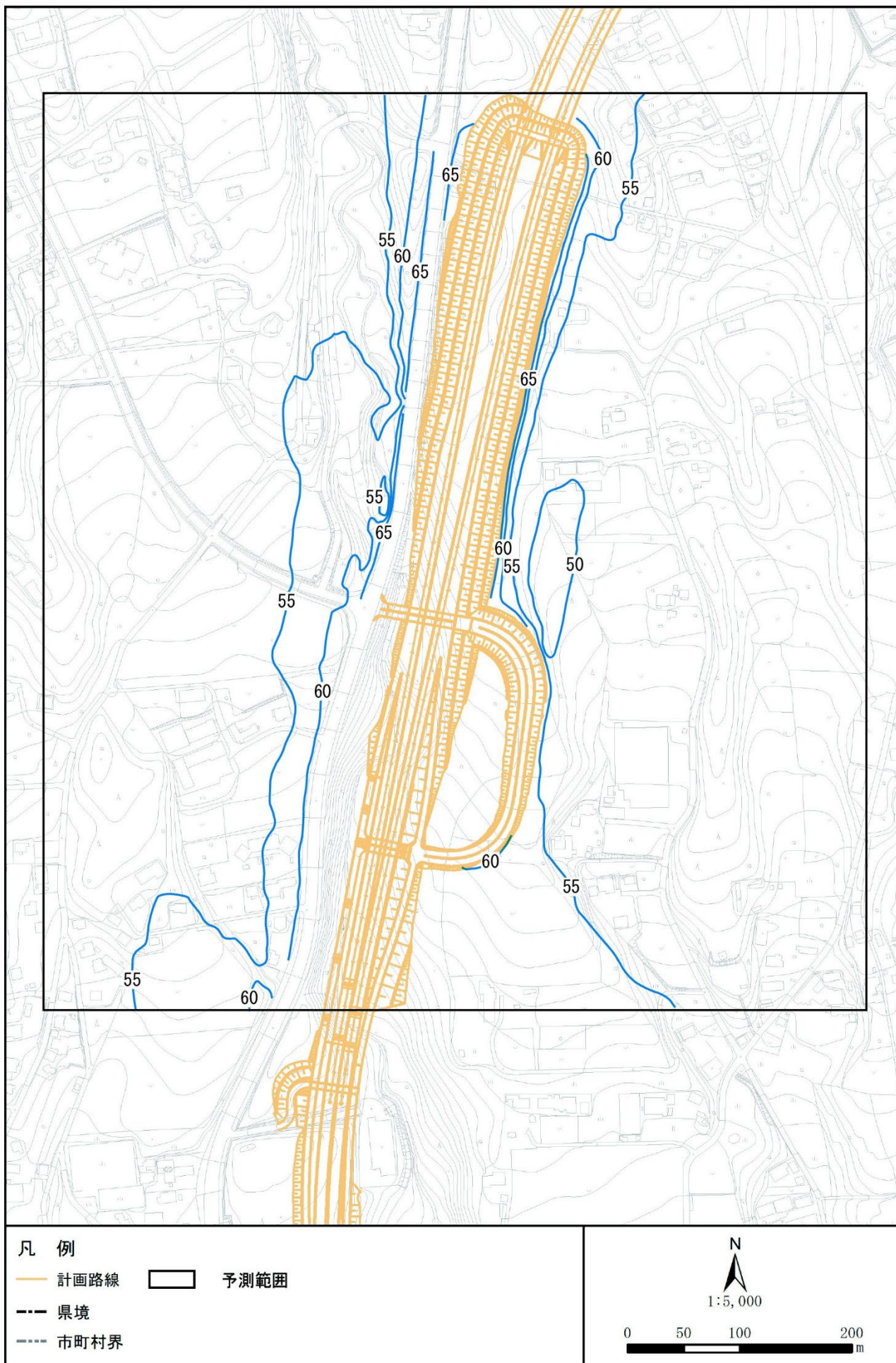
図 3.1-1 (13) 騒音分布図 (Y9. 高根町清里 3) 地上 1.2m 屋間
