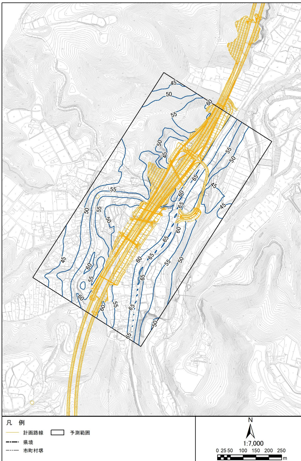
図 3.1-2 (16) 環境保全措置後の騒音分布図 (N5. 小海町豊里1) 地上 4.2m 夜間
