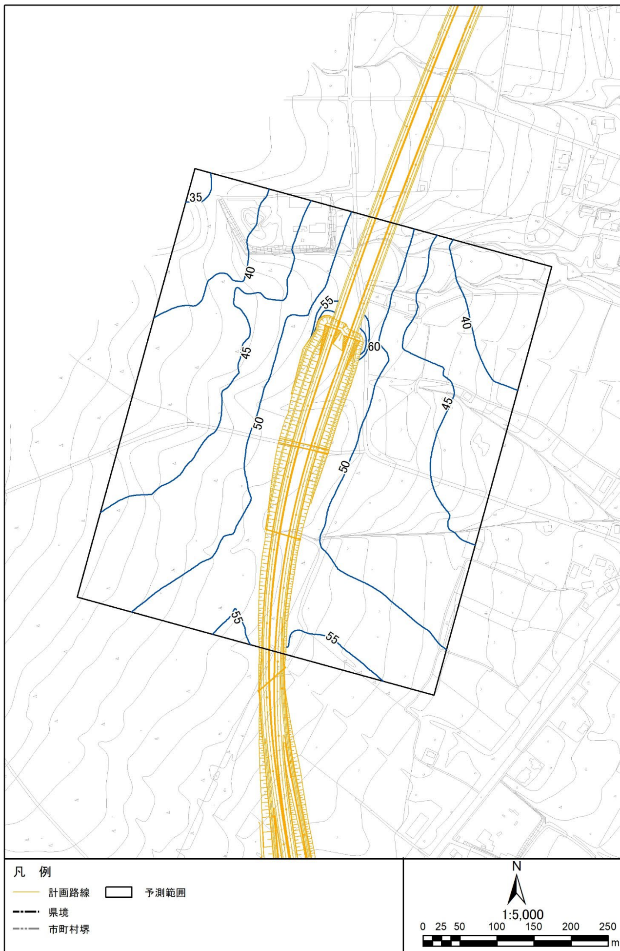
図 3.1-2 (9) 環境保全措置後の騒音分布図 (N2. 南牧村野辺山 2) 地上 1.2m 昼間
