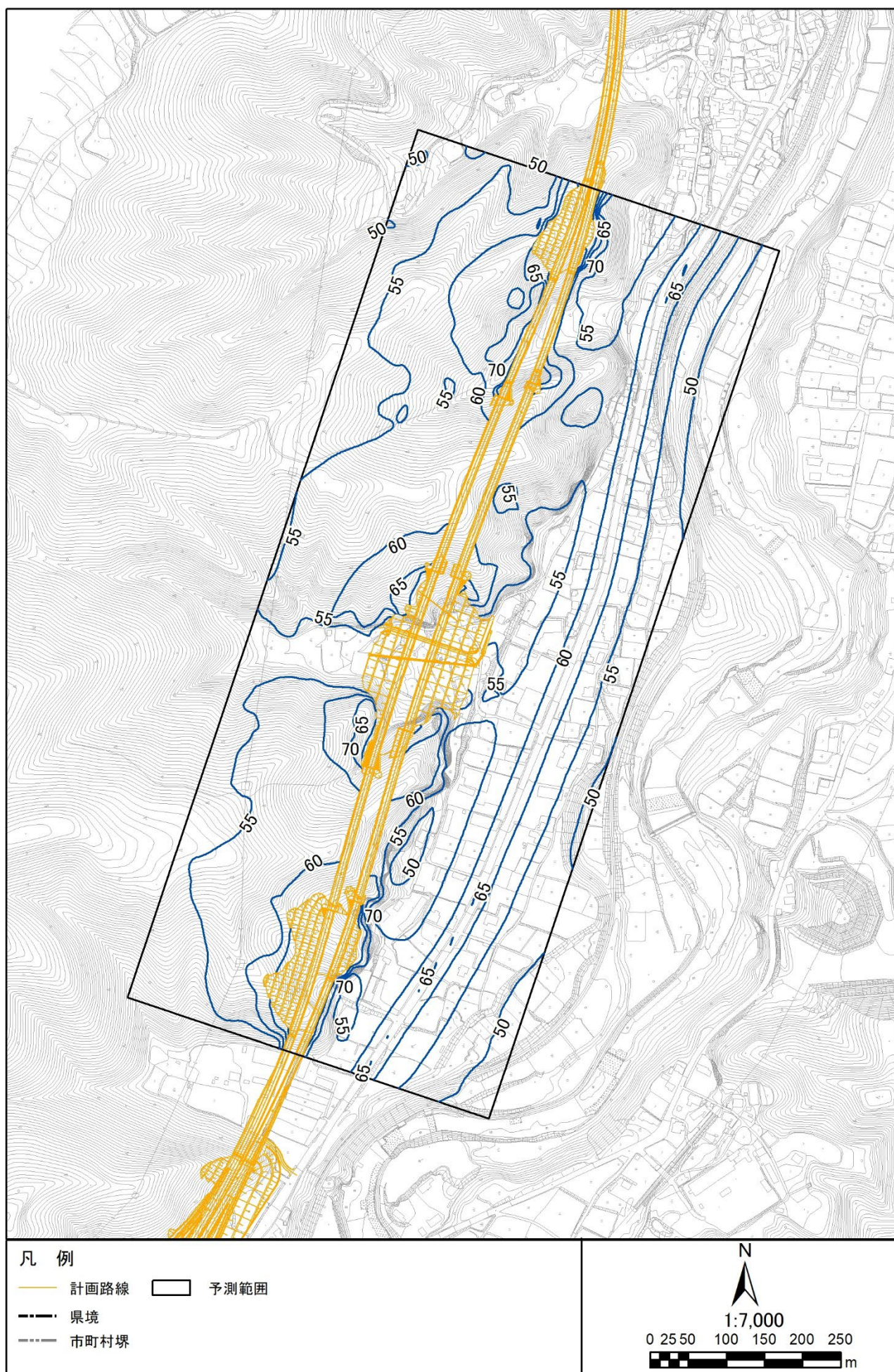
図 3.1-1 (32) 騒音分布図 (N6. 小海町豊里鎚掛1) 地上 4.2m 夜間
