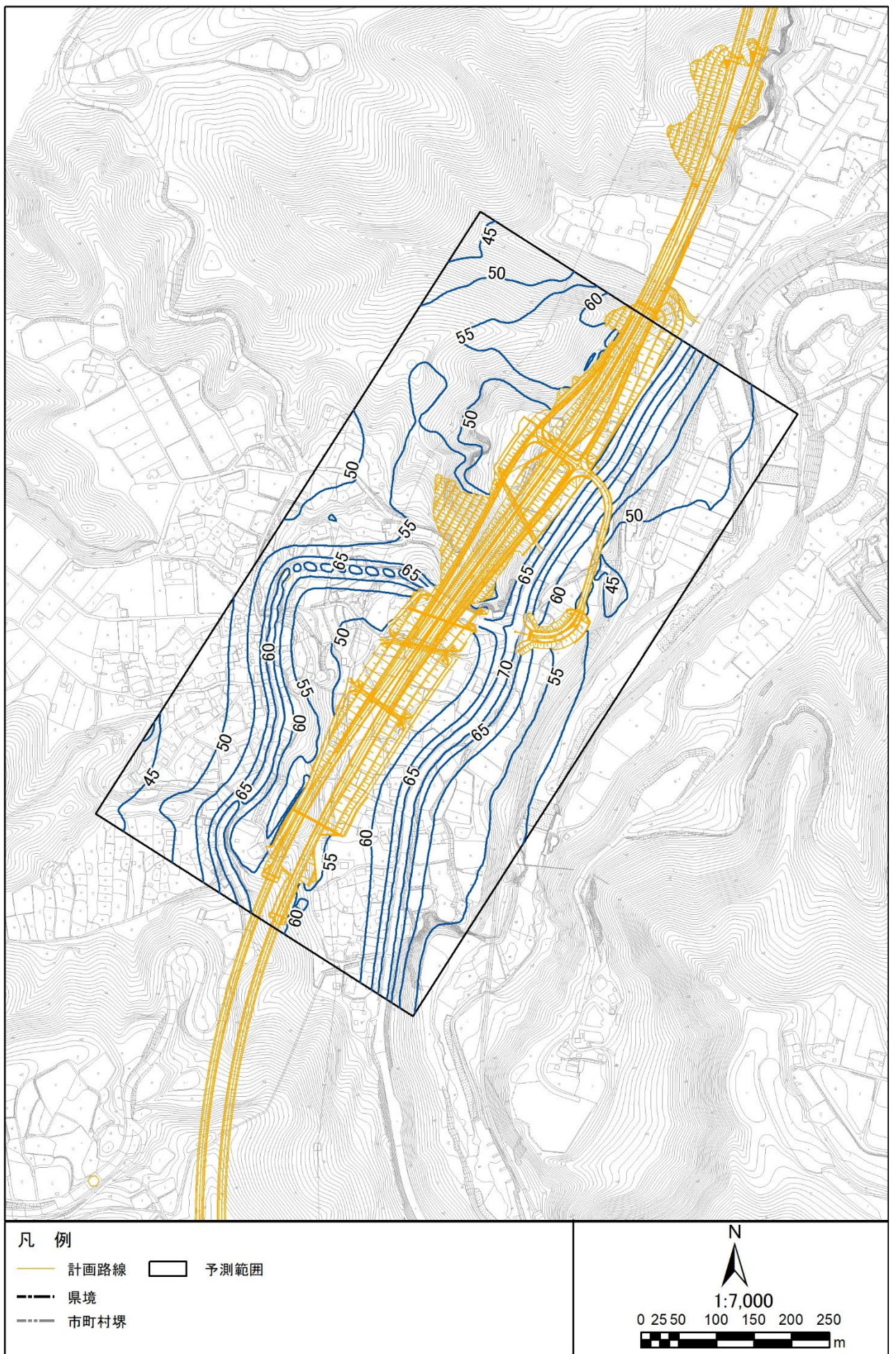
図 3.1-2 (13) 環境保全措置後の騒音分布図 (N5. 小海町豊里1) 地上 1.2m 昼間
