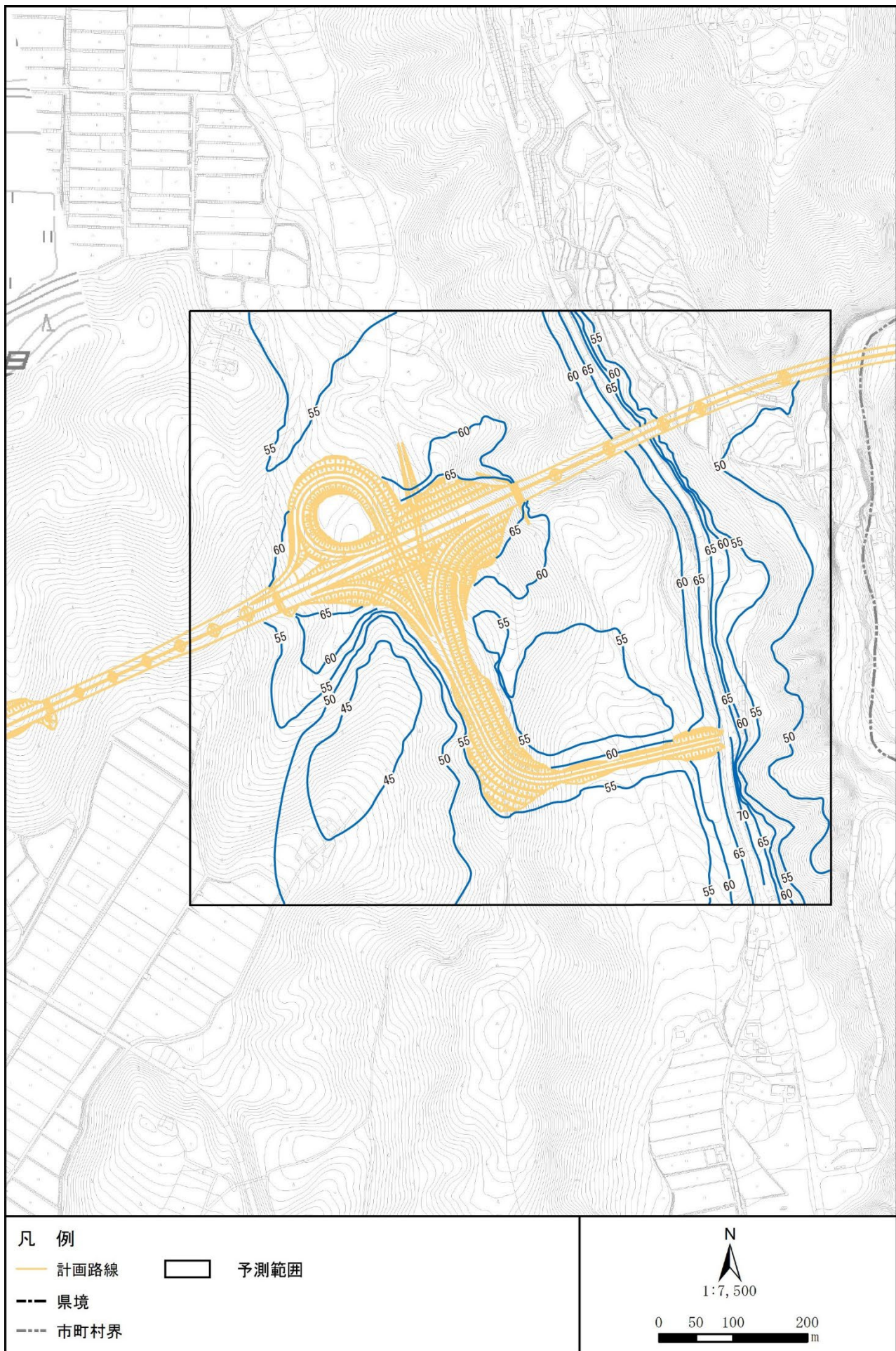
図 3.1-1 (6) 騒音分布図 (Y5. 高根町堤) 地上 4.2m 屋間
