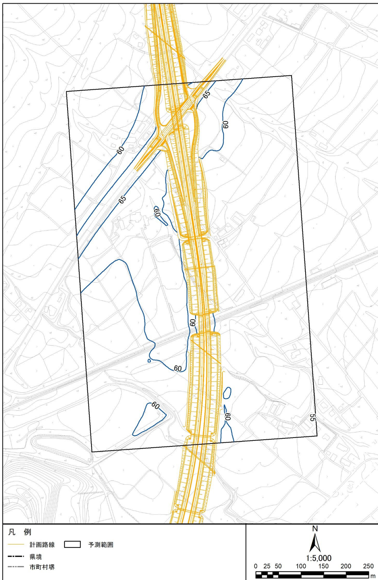
図 3.1-2 (6) 環境保全措置後の騒音分布図 (N1. 南牧村野辺山1) 地上 4.2m 昼間
