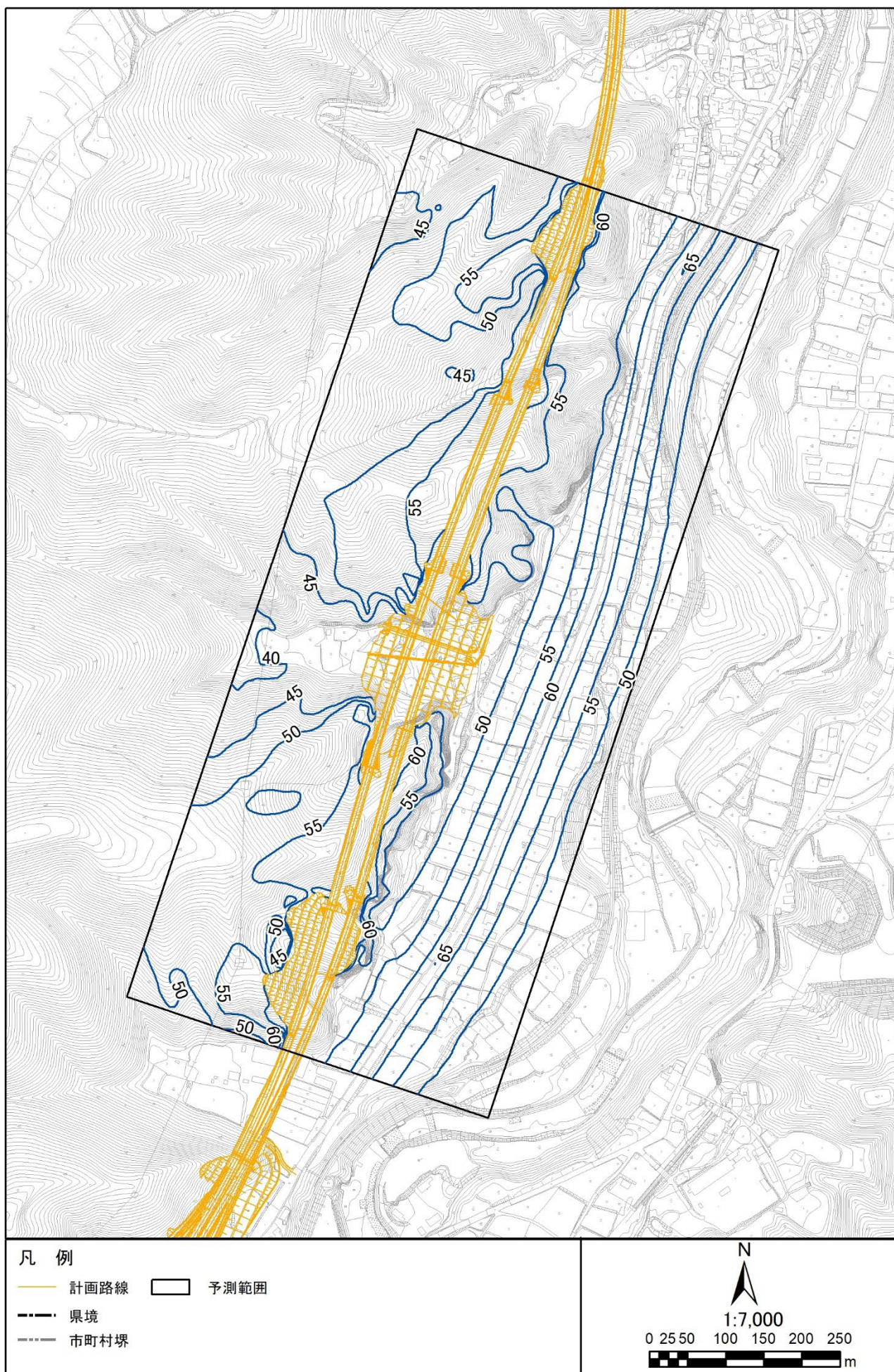
図 3.1-2 (20) 環境保全措置後の騒音分布図 (N6. 小海町豊里鎰掛 1) 地上 4.2m 夜間
