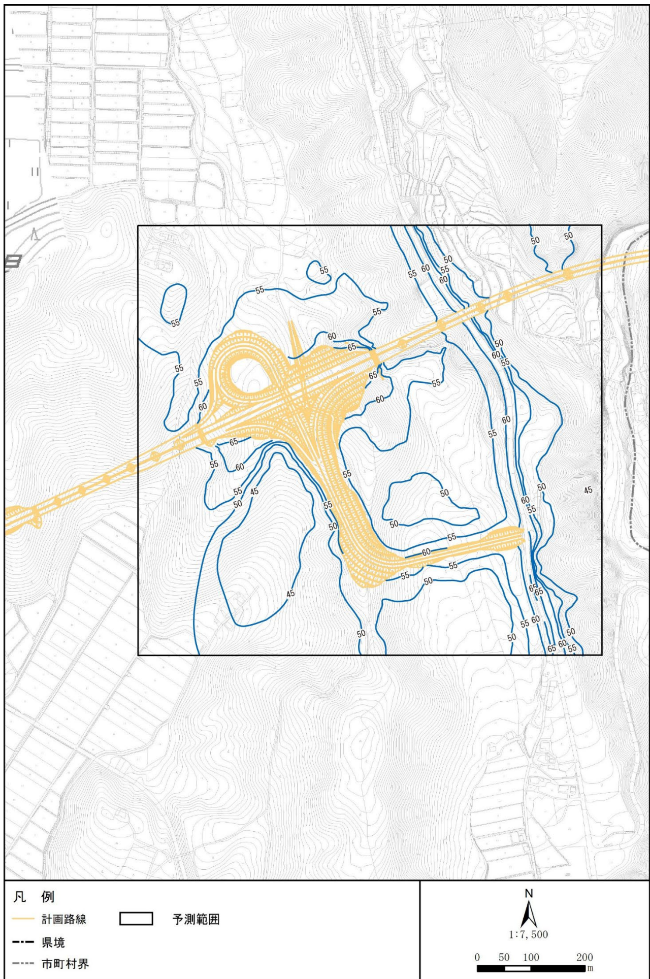
図 3.1-1 (8) 騒音分布図 (Y5. 高根町堤) 地上 4.2m 夜間
