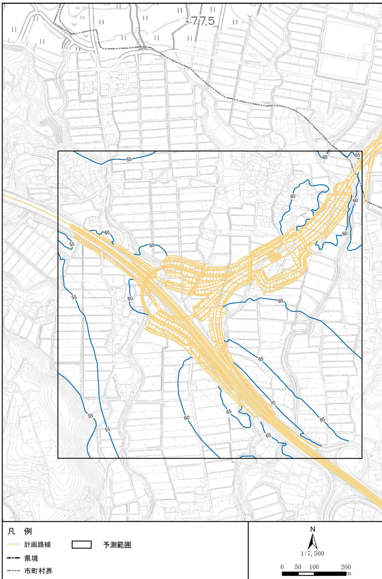
図 3.1-1 (2) 騒音分布図 (Y1. 長坂町大八田) 地上 4.2m 昼間
