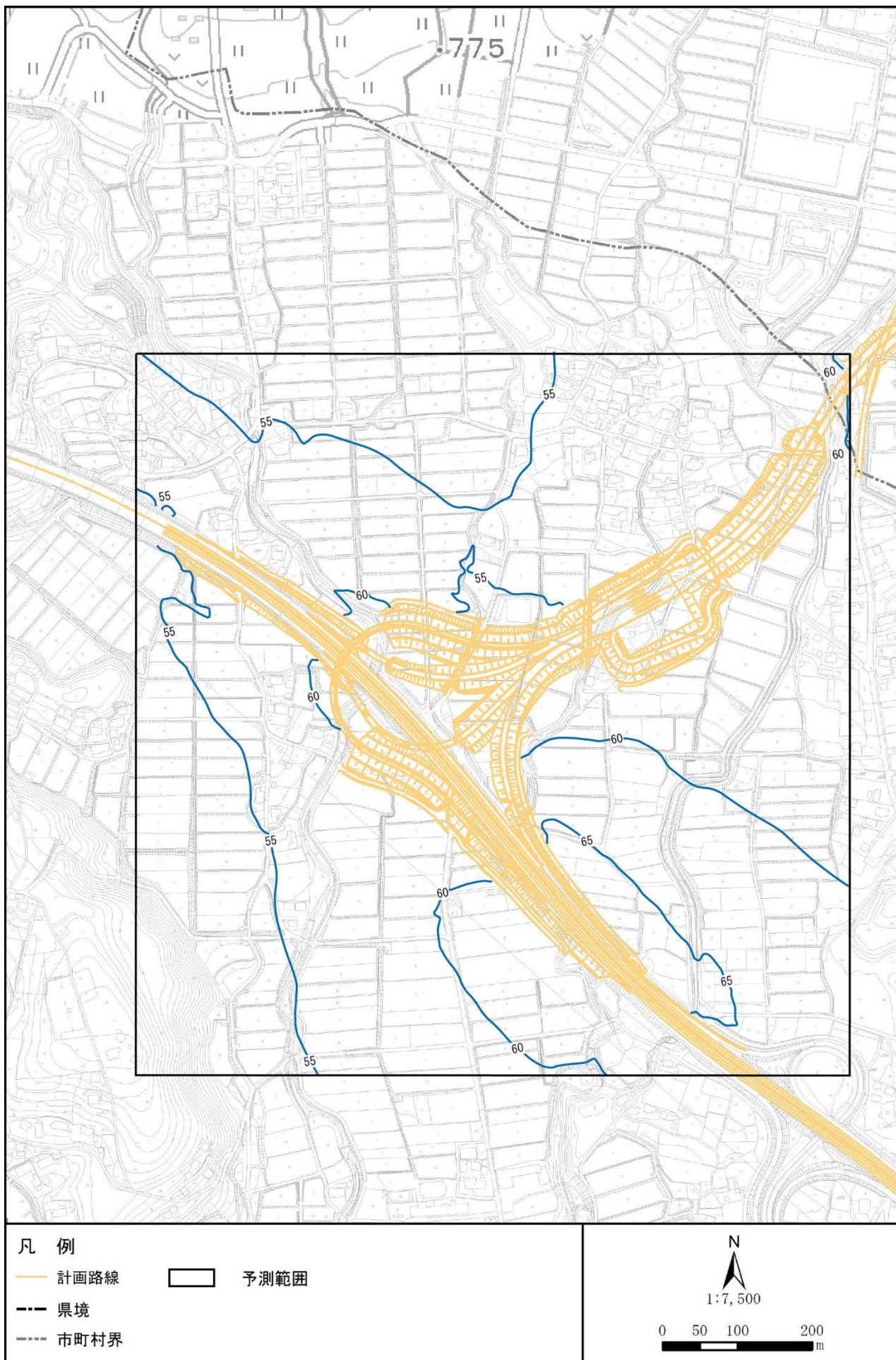
図 3.1-1 (3) 騒音分布図 (Y1. 長坂町大八田) 地上 1.2m 夜間
