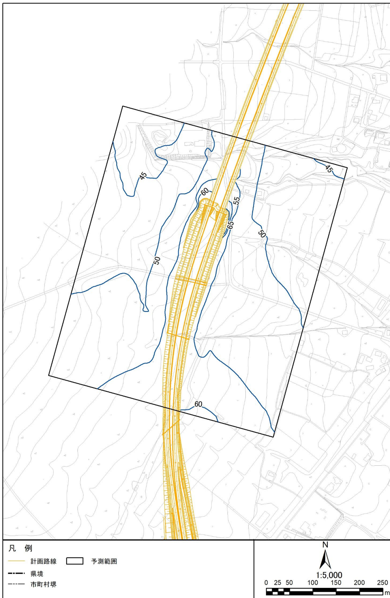
図 3.1-2 (10) 環境保全措置後の騒音分布図 (N2. 南牧村野辺山 2) 地上 4.2m 昼間
