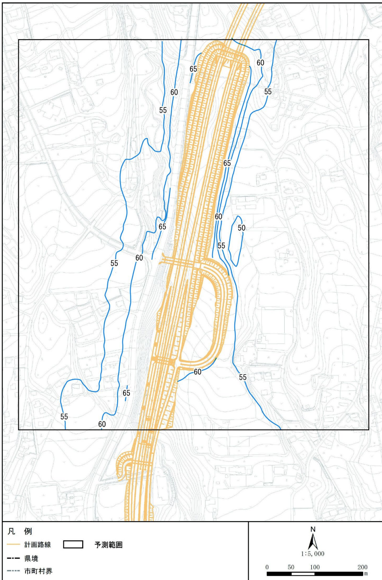
図 3.1-1 (14) 騒音分布図 (Y9. 高根町清里 3) 地上 4.2m 屋間
