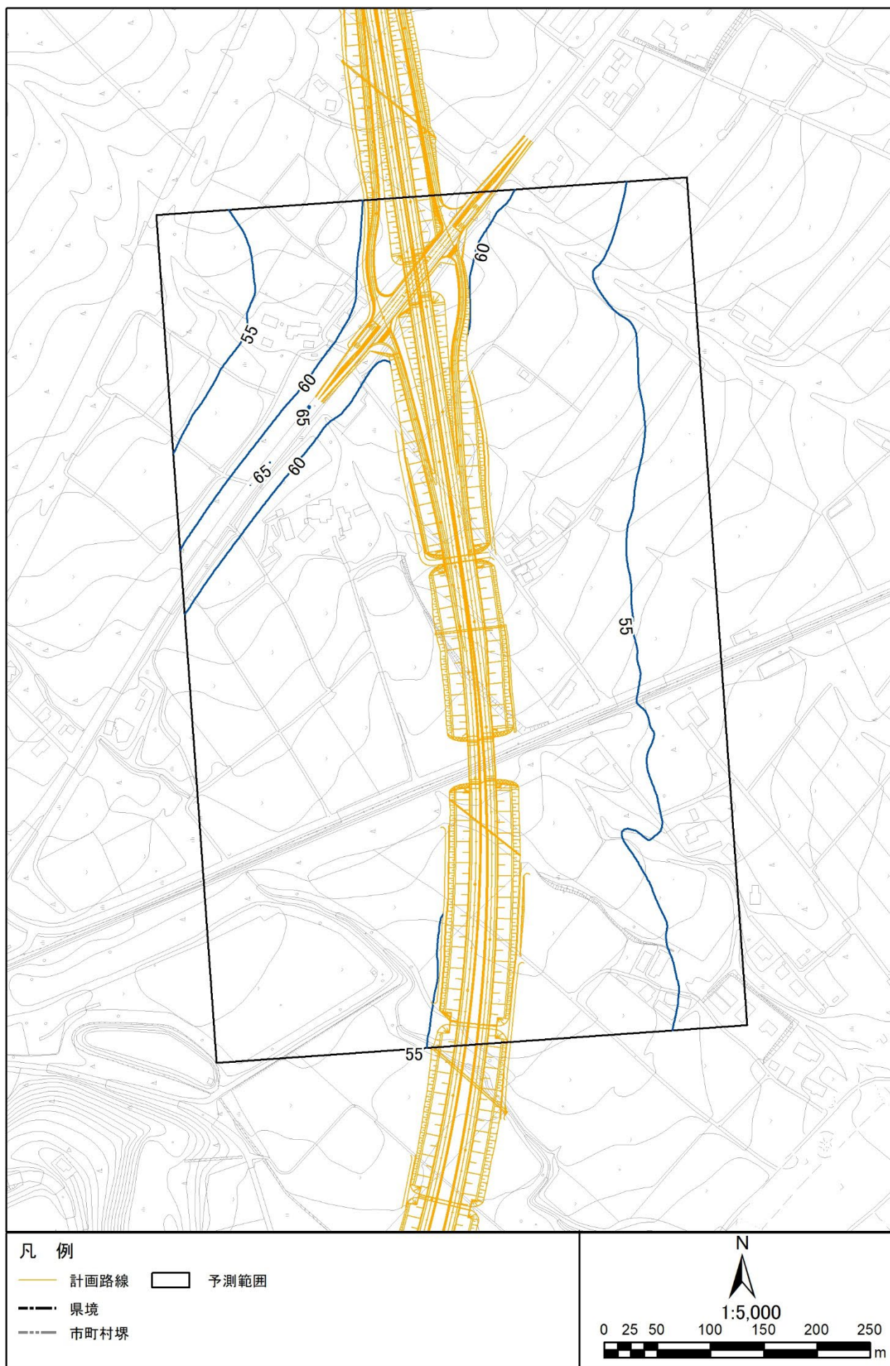
図 3.1-2 (8) 環境保全措置後の騒音分布図 (N1. 南牧村野辺山 1) 地上 4.2m 夜間
