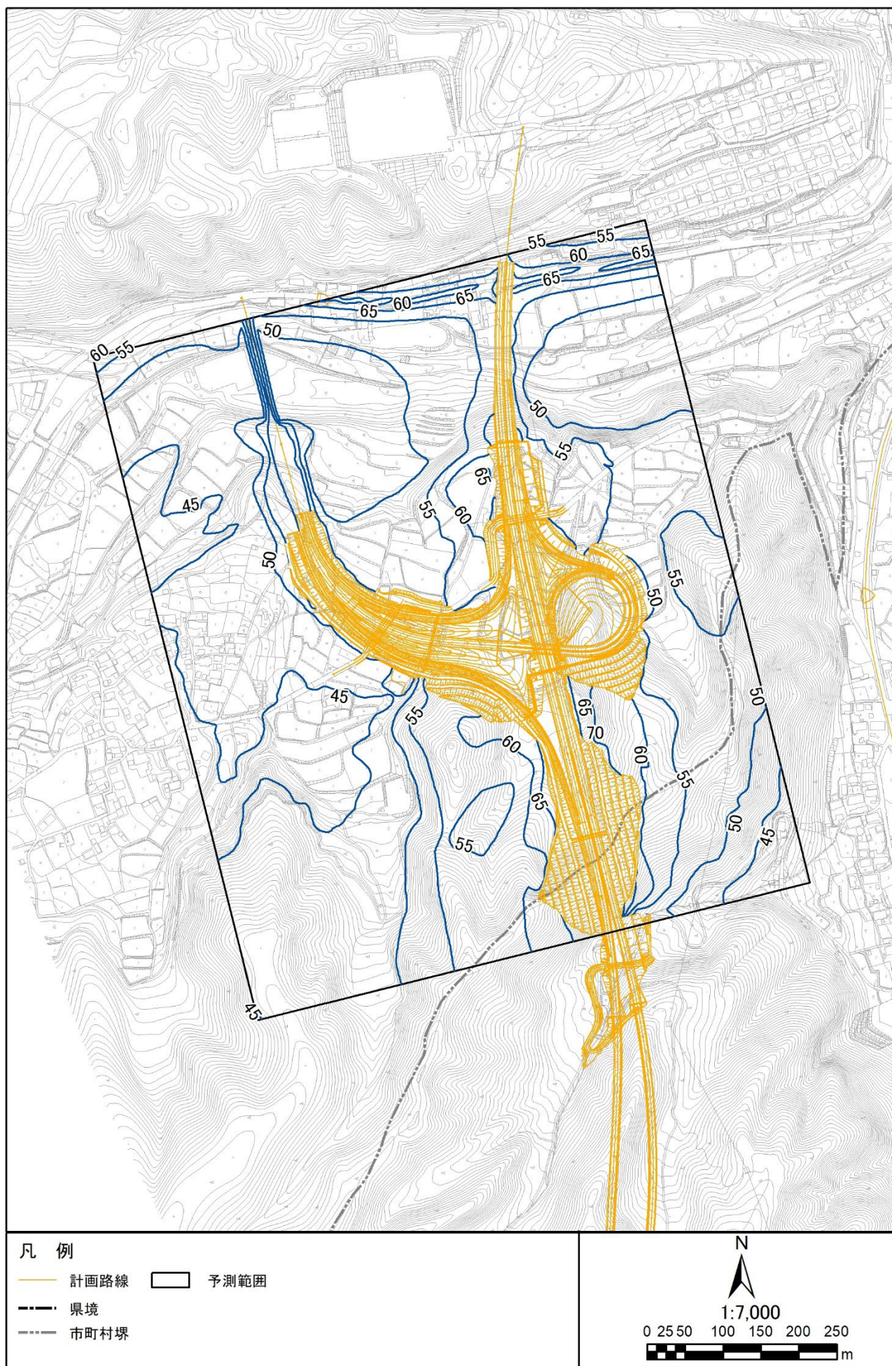
図 3.1-1 (35) 騒音分布図 (N9. 佐久穂町千代里) 地上 1.2m 夜間
