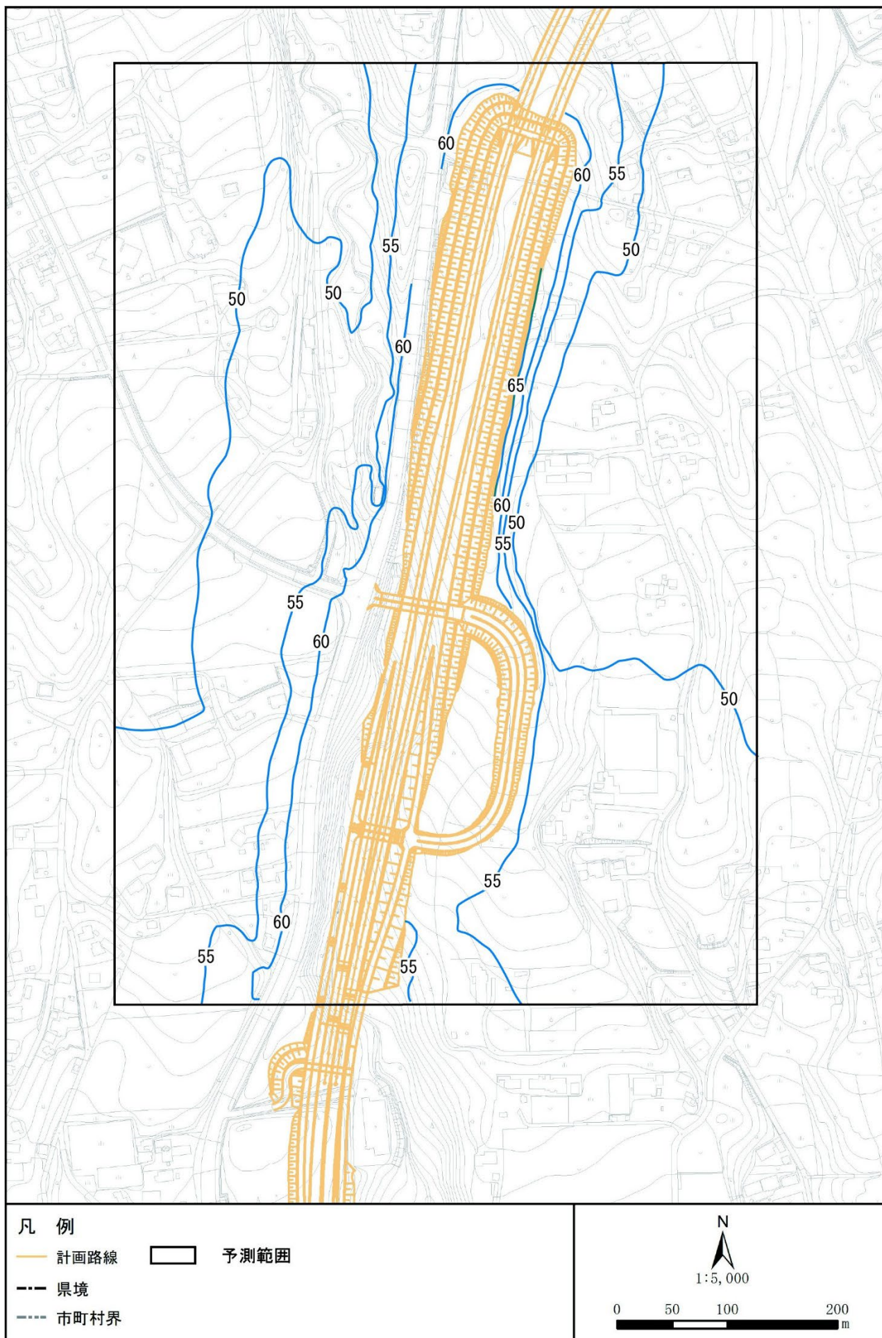
図 3.1-2 (4) 環境保全措置後の騒音分布図 (Y9. 高根町清里 3) 地上 4.2m 夜間
