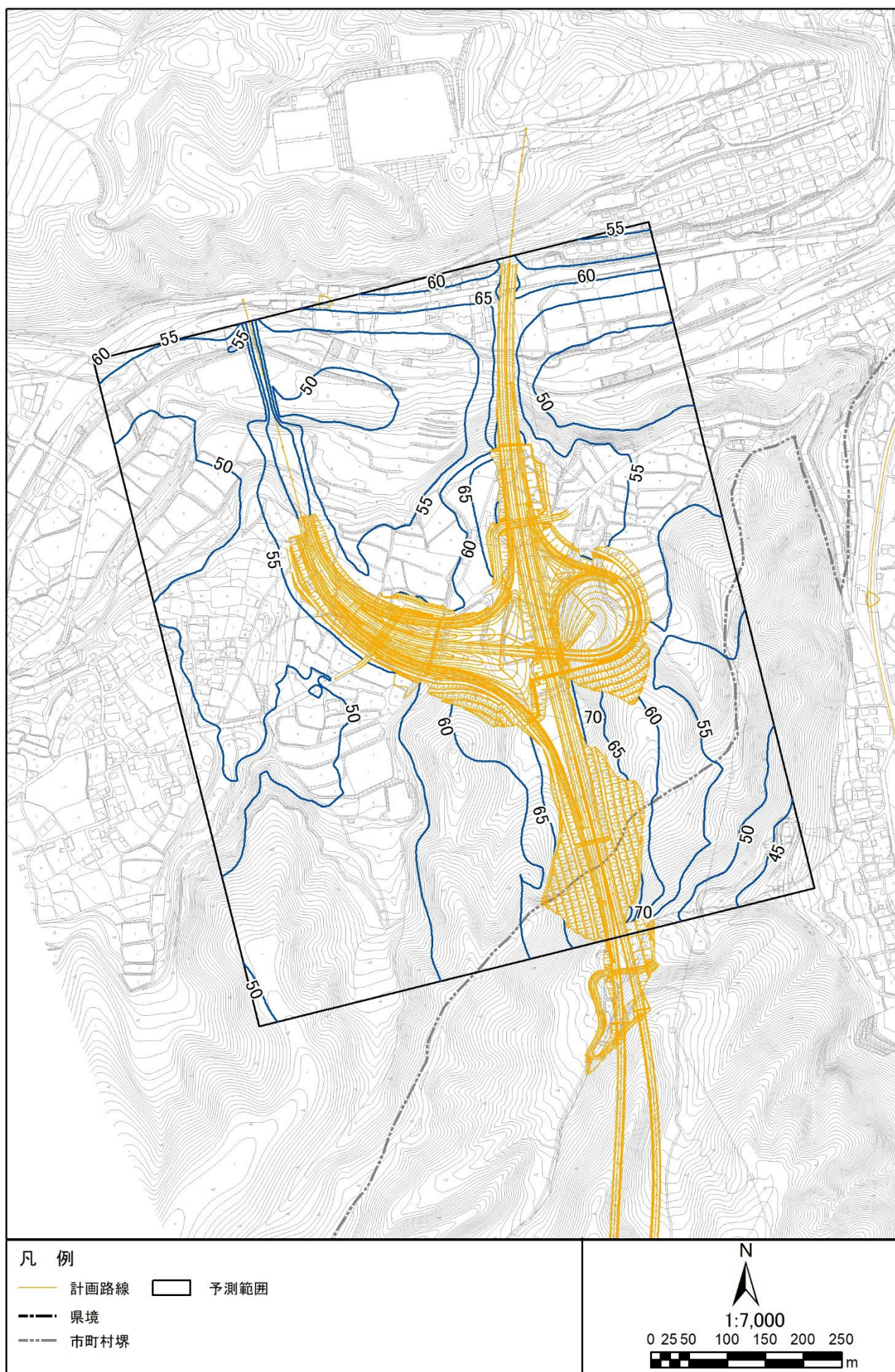
図 3.1-1 (36) 騒音分布図 (N9. 佐久穂町千代里) 地上 4.2m 夜間
