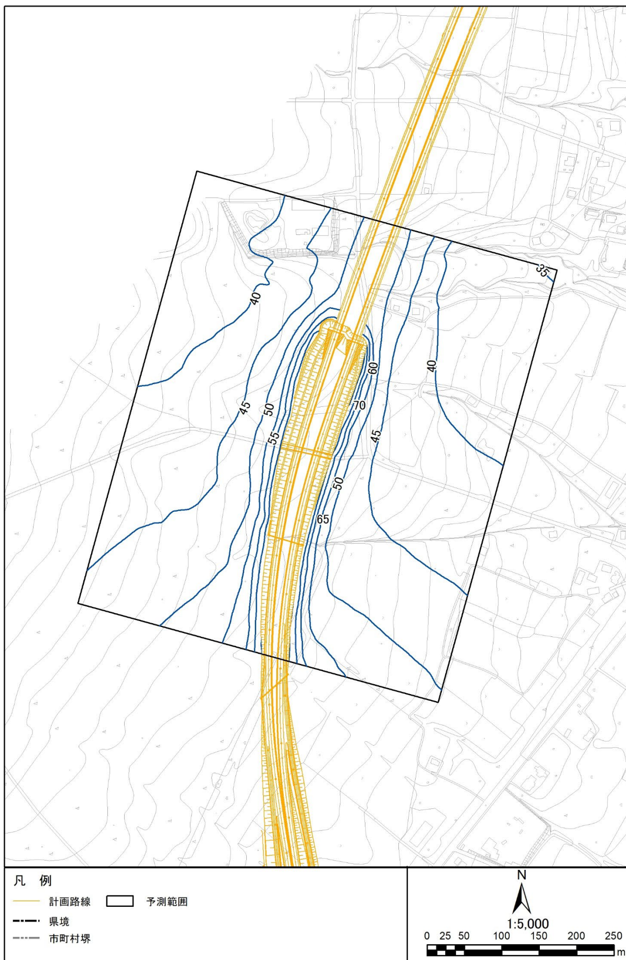
図 3.1-1 (23) 騒音分布図 (N2. 南牧村野辺山2) 地上 1.2m 夜間
