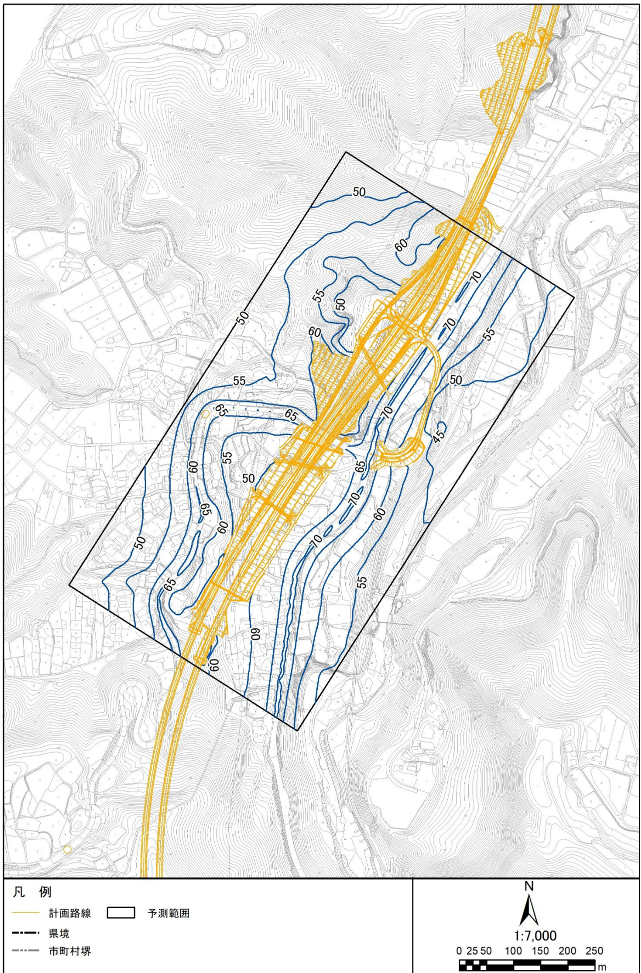
図 3.1-2 (14) 環境保全措置後の騒音分布図 (N5. 小海町豊里 1) 地上 4.2m 昼間
