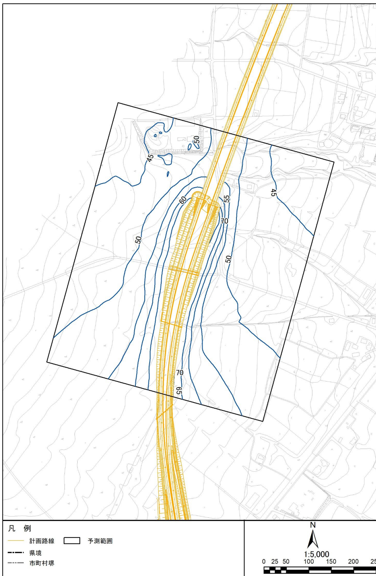
図 3.1-1 (24) 騒音分布図 (N2. 南牧村野辺山 2) 地上 4.2m 夜間
