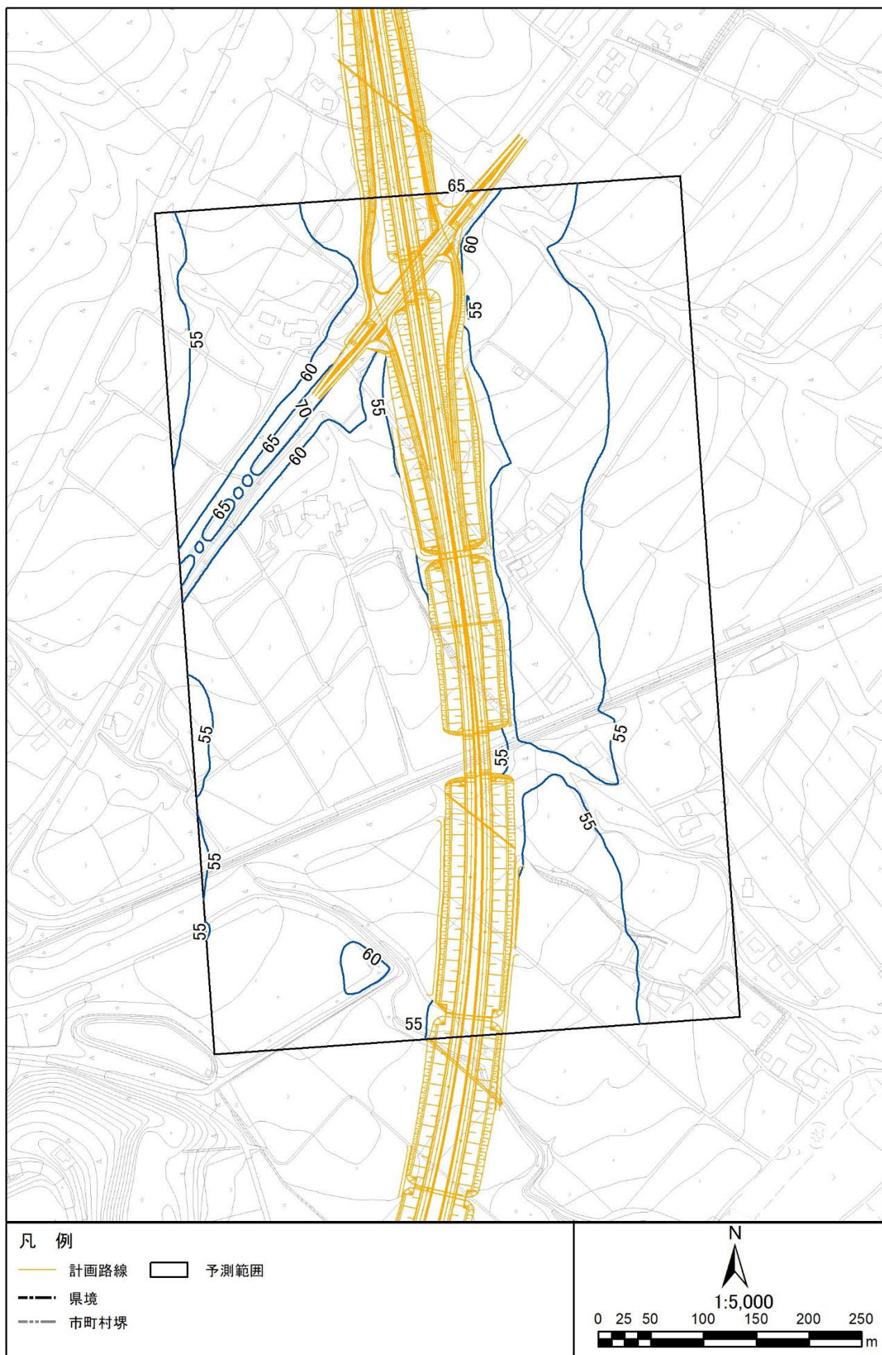
図 3.1-1 (19) 騒音分布図 (N1. 南牧村野辺山 1) 地上 1.2m 夜間
