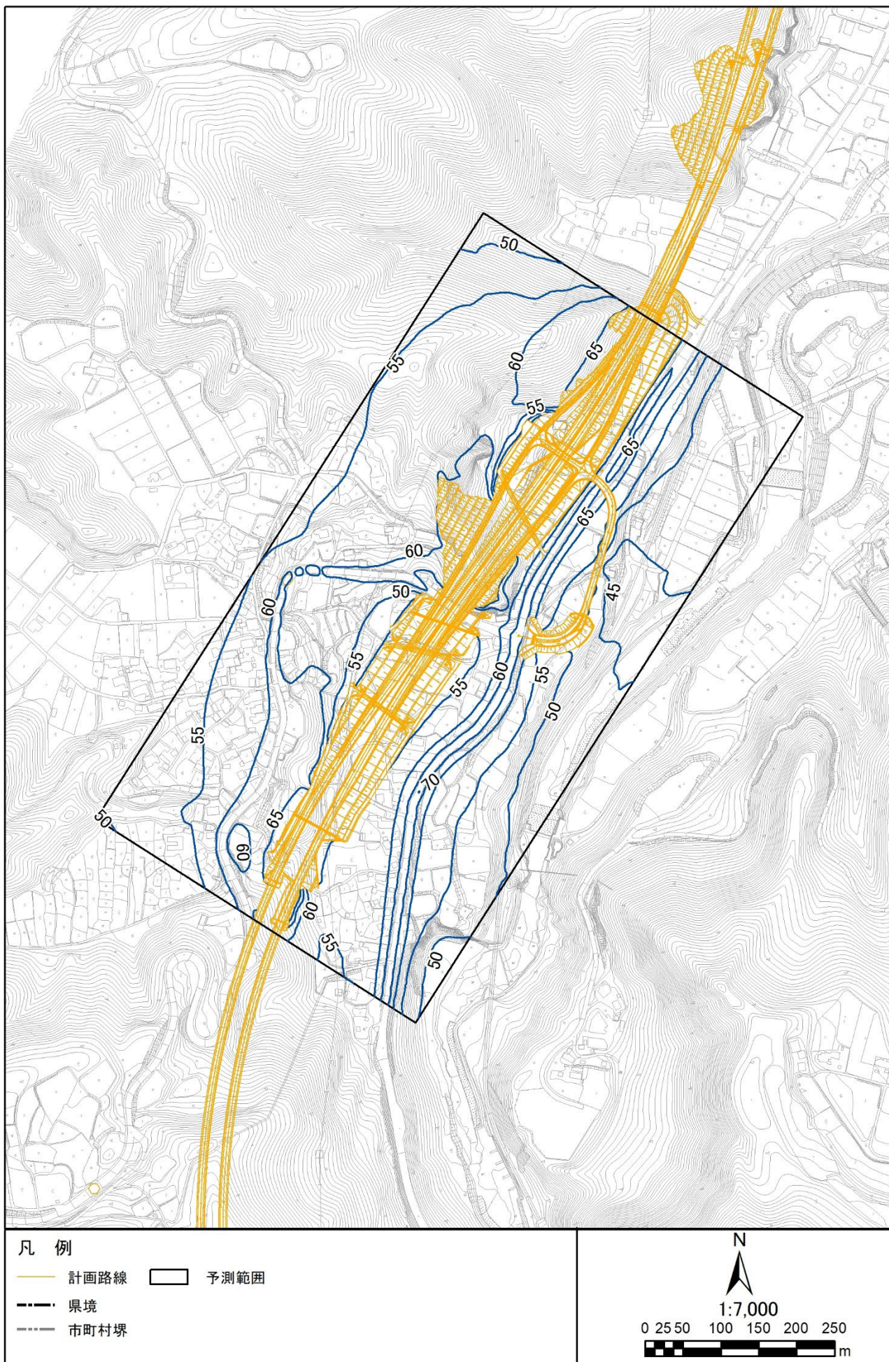
図 3.1-1 (27) 騒音分布図 (N5, 小海町豊里1) 地上 1.2m 夜間
