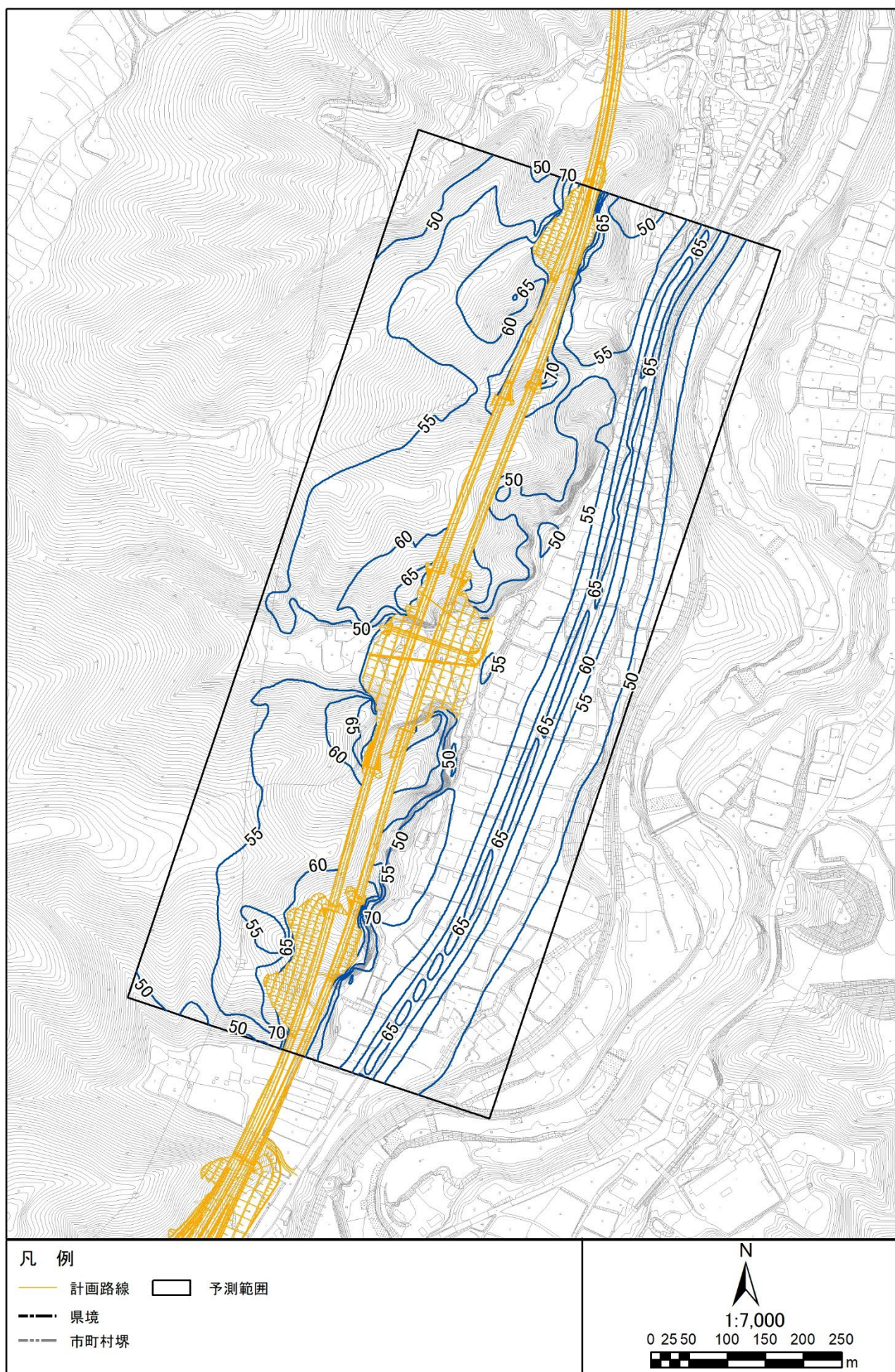
図 3.1-1 (31) 騒音分布図 (N6. 小海町豊里鎚掛1) 地上 1.2m 夜間
