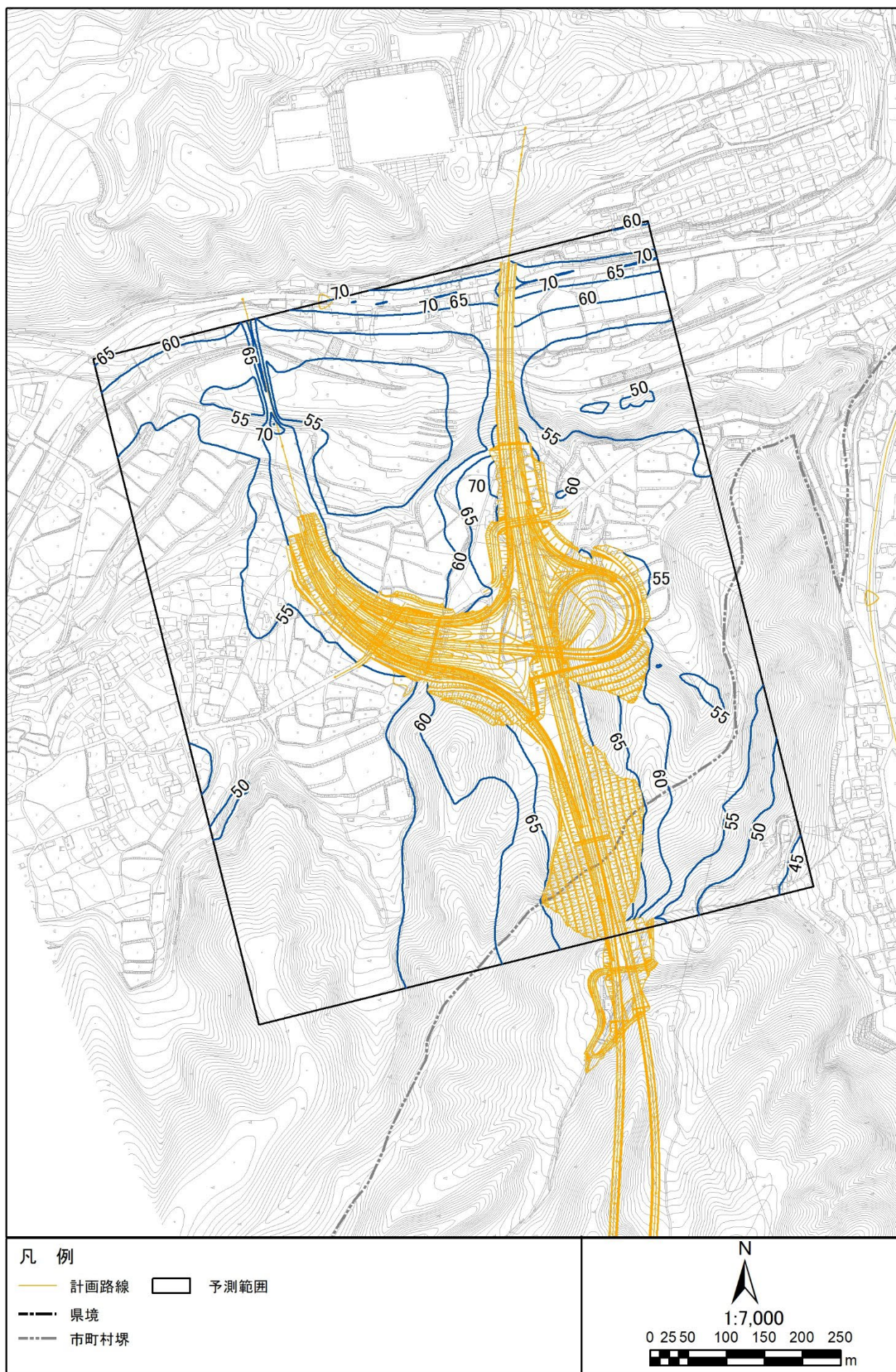
図 3.1-1 (34) 騒音分布図 (N9. 佐久穂町千代里) 地上 4.2m 昼間
