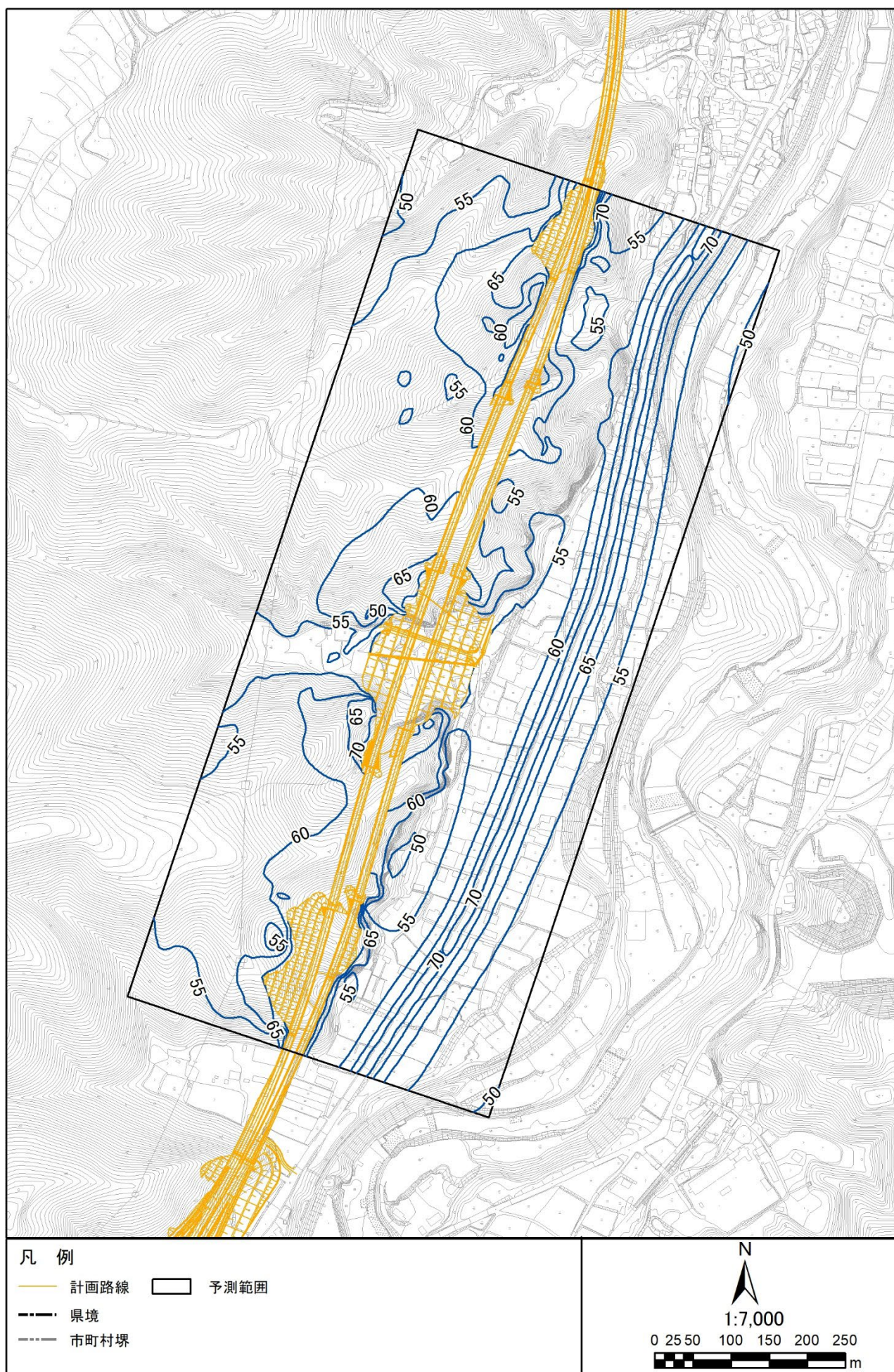
図 3.1-1 (29) 騒音分布図 (N6. 小海町豊里鎰掛 1) 地上 1.2m 昼間
