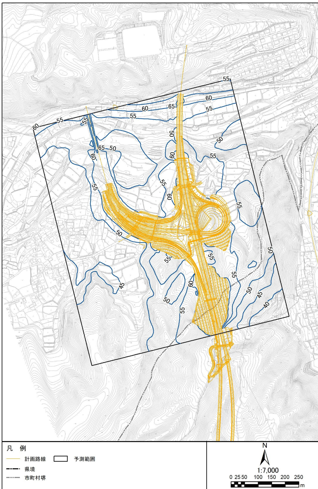
図 3.1-2 (24) 環境保全措置後の騒音分布図 (N9. 佐久穂町千代里) 地上 4.2m 夜間
