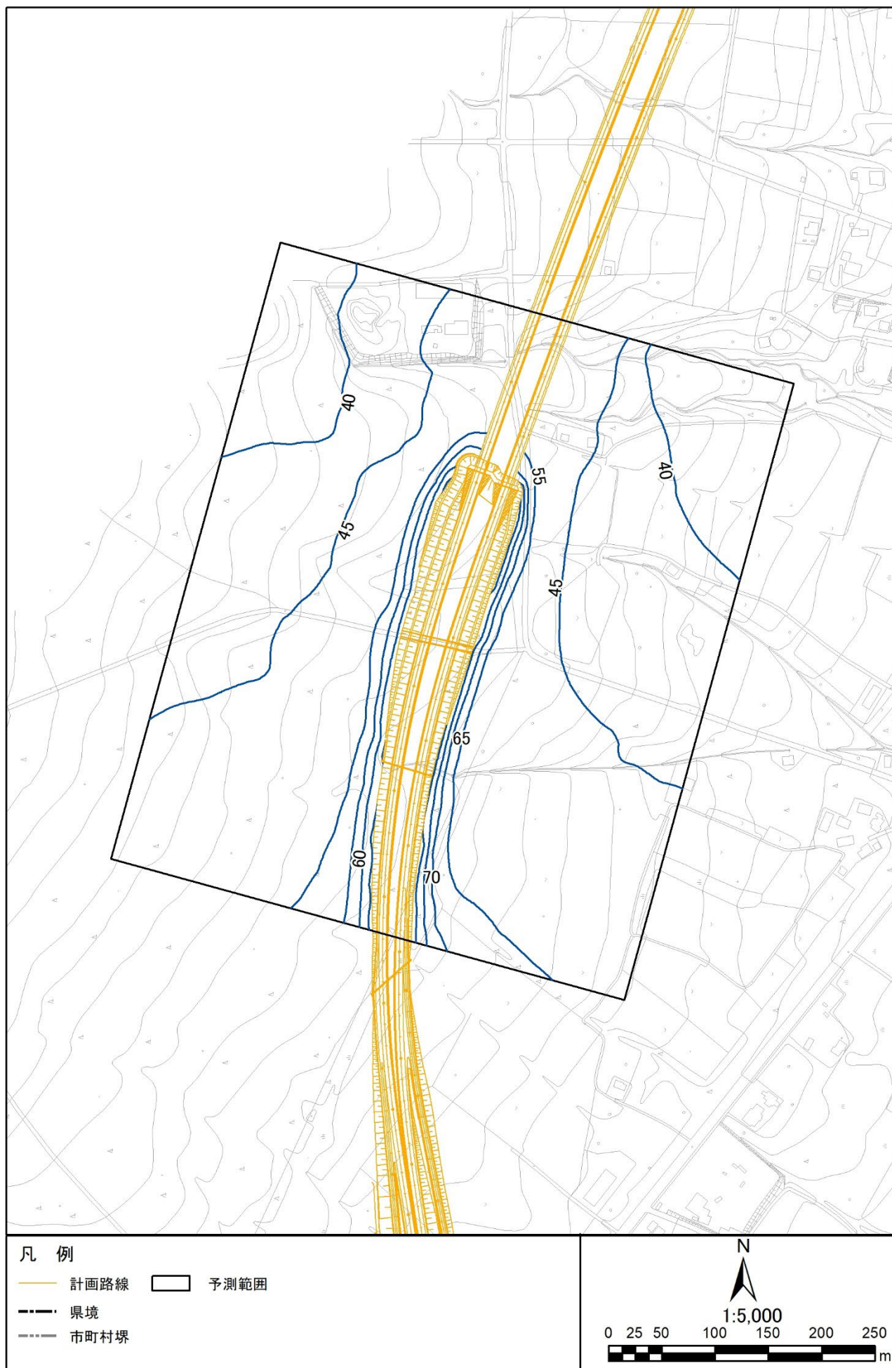
図 3.1-1 (21) 騒音分布図 (N2. 南牧村野辺山 2) 地上 1.2m 昼間
