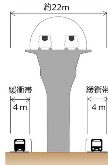
リニア本線用地の緩衝帯での走行イメージ
