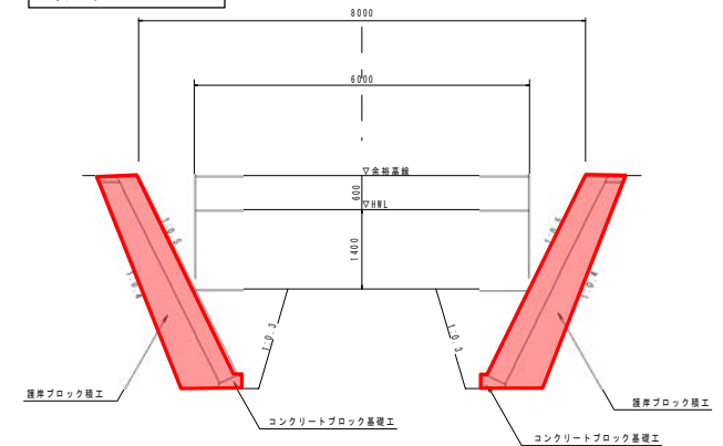
標準断面図
